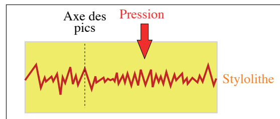
Schéma de la formation d'un joint stylolithique.
