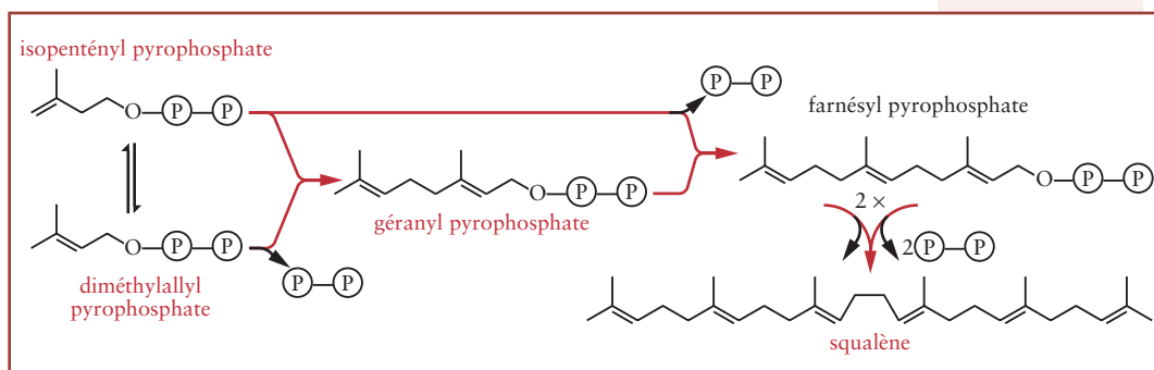
Figure 19.6 Étape 3 : formation du squalène.
