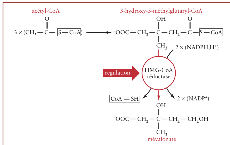
Figure 19.4 Étape 1 : formation du mévalonate.
