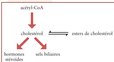
Figure 19.2 Relations métaboliques du cholestérol.
