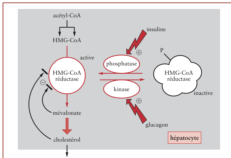
Figure 19.8 Régulation à court terme de la biosynthèse du cholestérol.
