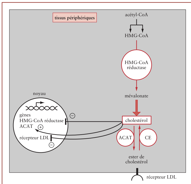
Figure 19.9 Régulation à long terme de la biosynthèse du cholestérol.
