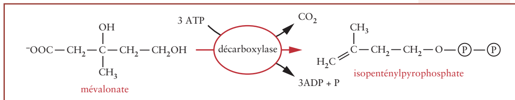
Figure 19.5 Étape 2 : formation de l'isopentényl-pyrophosphate.
